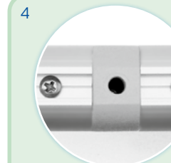
Nachträglich verändern: einfach Profilrohr trennen und Verbinder Ihrer Wahl einbauen, z. B. Linienverbinder RVS/LV
