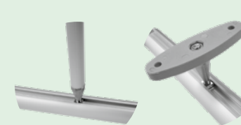
Verankerung an Profilschiene: mittels Vierkantenmutter auf der ganzen Strecke möglich; Für verstellbare Deckenstütze RVS/DS oder mit Deckenhalter RVS/DH. Max. Abstand: 2 m.
