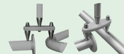
Abstandhalter: RVS/AH für Bogen und T-Lösung.
