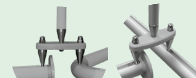
Système de pont: RVS/AH pour les courbes ou solutions en „T“
