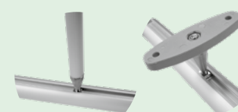
Ancrage sur rail profilé : possible à l'aide d'écrous carrés
