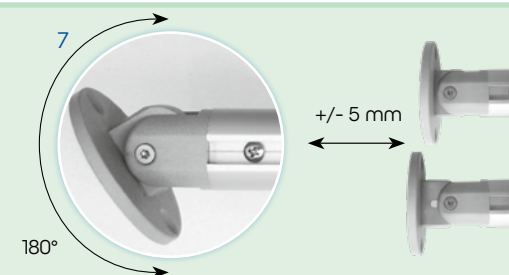
Murs inclinés, angles aigus : le raccord mural Vario RVS/WAV compense les asymétries jusqu'à 180° ainsi que les différences de longueurs jusqu'à +/- 5 mm
